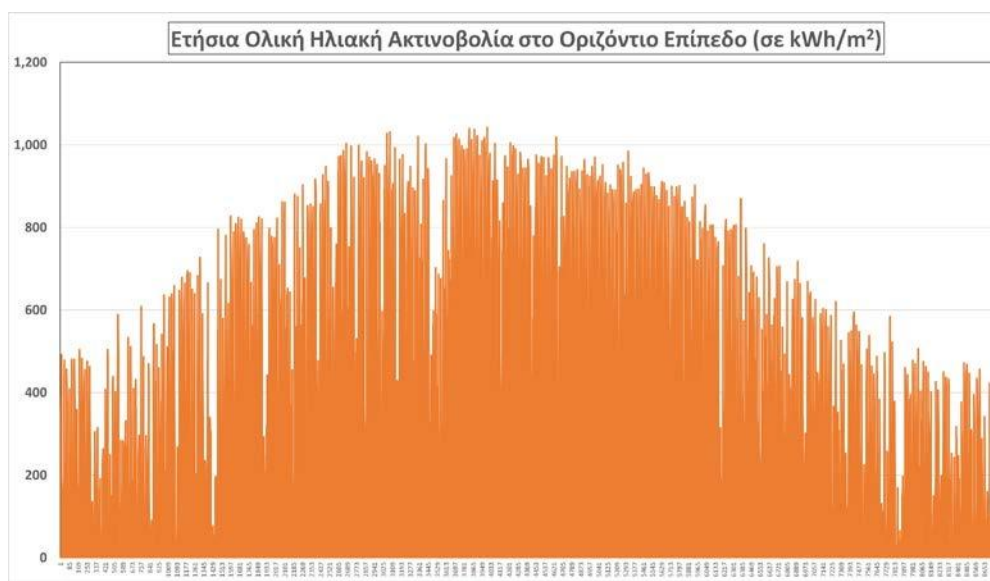
Εικόνα 1: Ωριαία μεταβολή ηλιακής ακτινοβολίας στο οριζόντιο επίπεδο για χρονικό διάστημα ενός έτους (μετρήσεις ηλιακής ακτινοβολίας στο χώρο της Π2).
